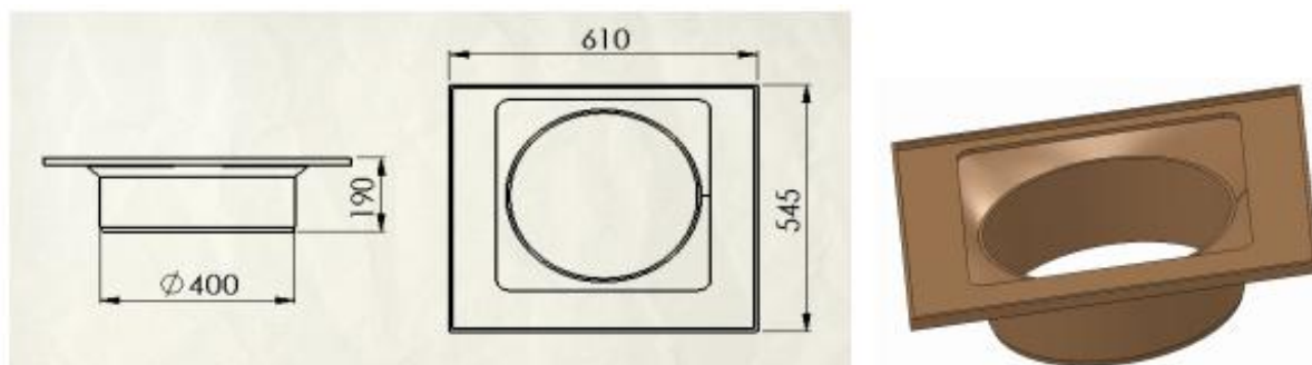
Piesa sprijin pentru gratar fonta clasa D400
