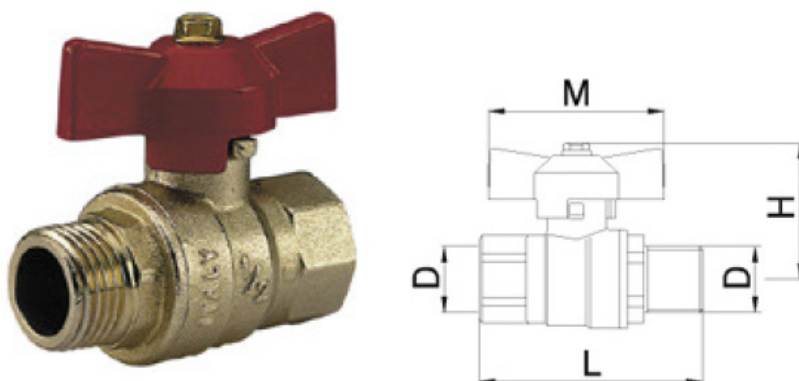
Art.434B. Robinet cu sfera cu trecere totala cu racord MF PN25, fluture
