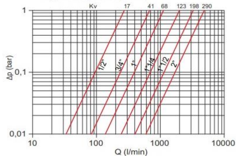
Digrama debit/pierderi de presiune
