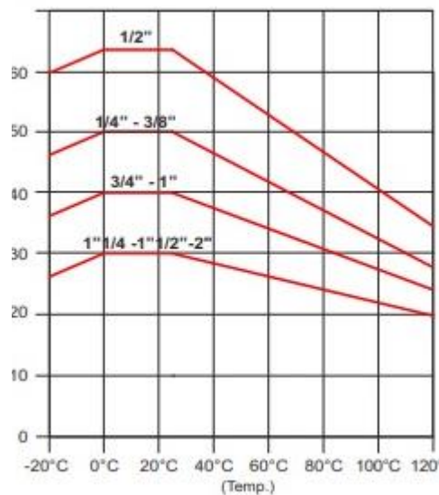
grama Presiune / temperatura
